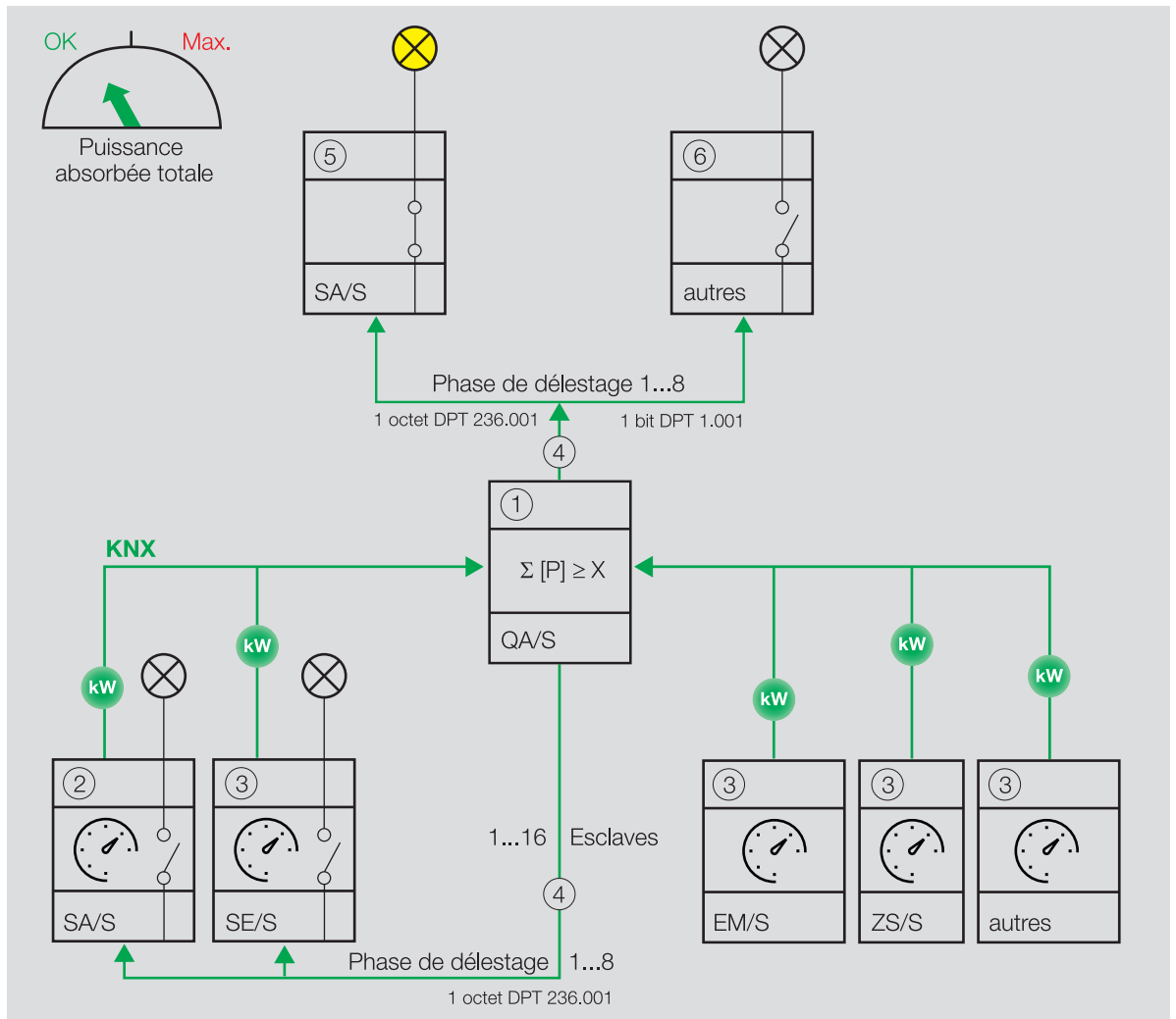
Fig. 18: Le maître diminue le niveau de déconnexion de charge.
