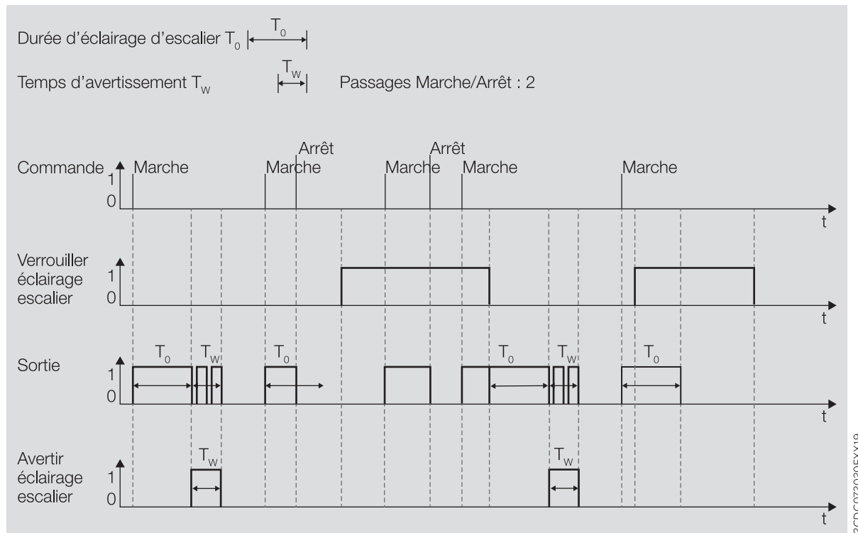
Fig. 20: Prolonger la durée d'éclairage escalier (réarmer/pomper)
