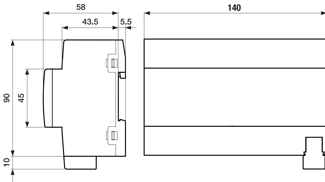
Fig. 8: Plan coté
