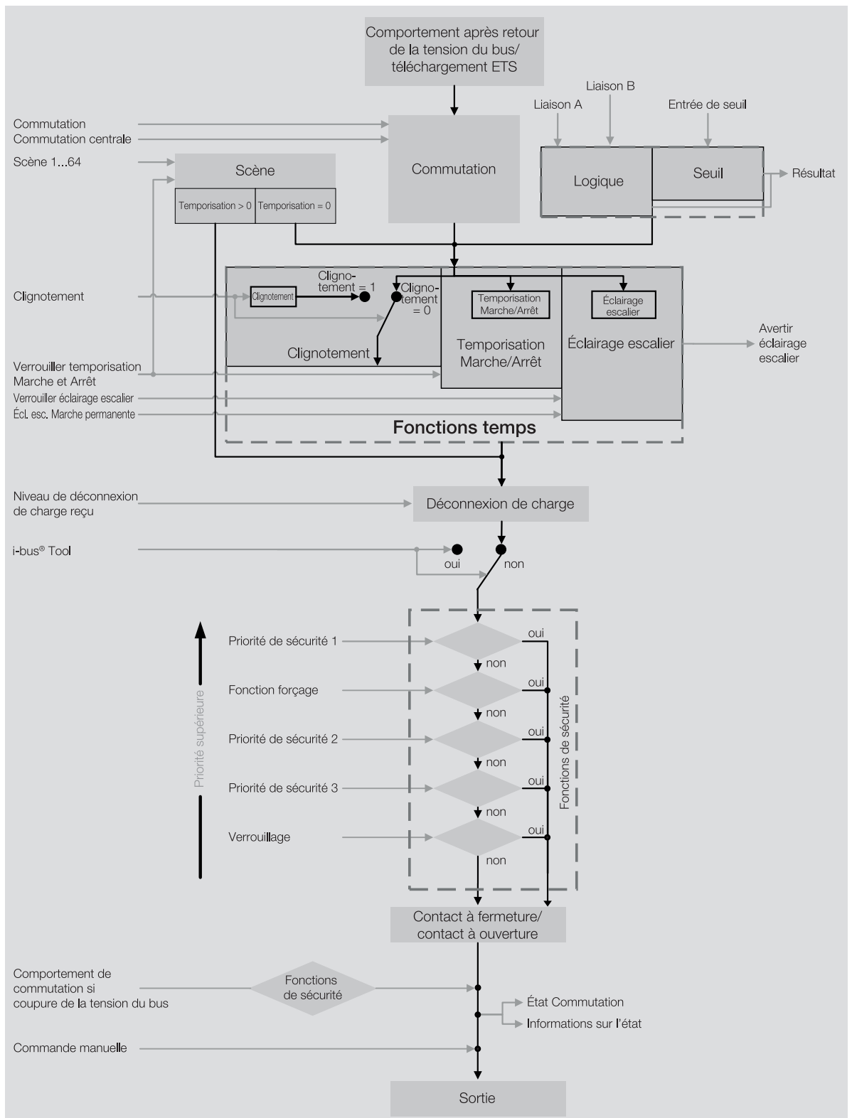
Fig. 13: Schéma des fonctions du module de commutation
