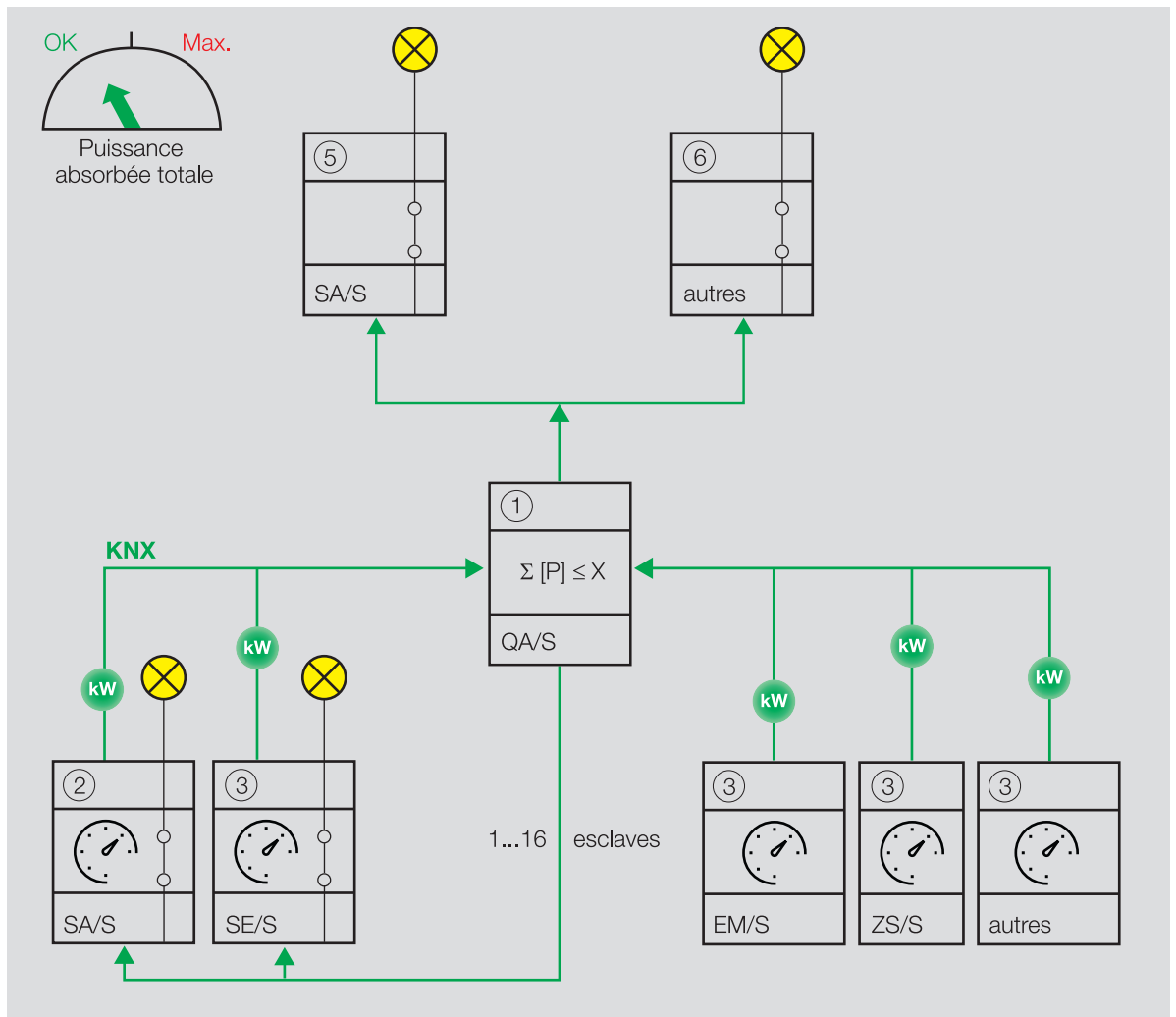
Fig. 14: Le maître reçoit des valeurs de puissance.
