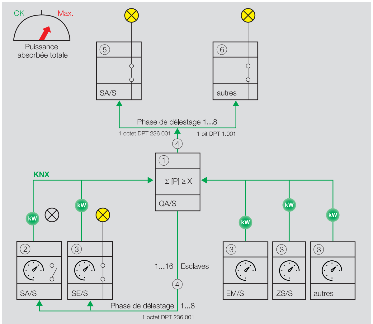
Fig. 16: Les esclaves reçoivent les niveaux de déconnexion de charge.
