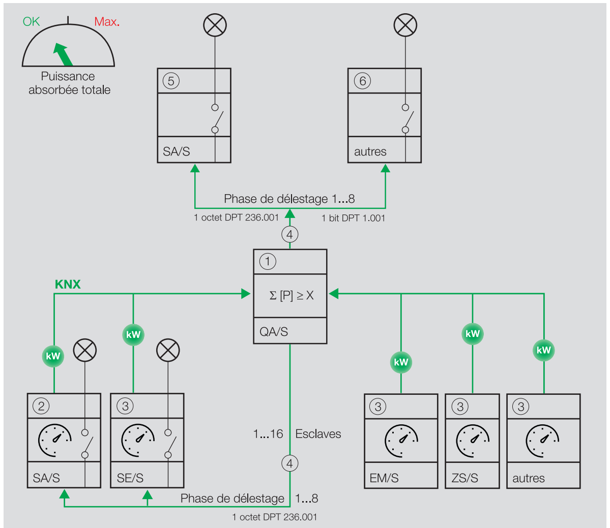
Fig. 17: Le maître augmente le niveau de déconnexion de charge.
