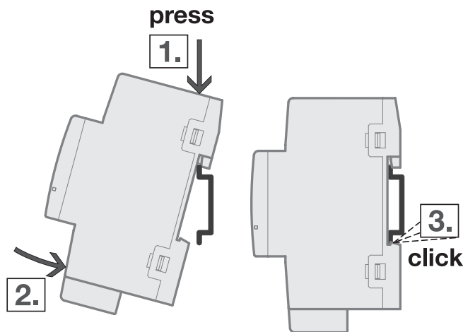
Fig. 21: Montage sur le rail
