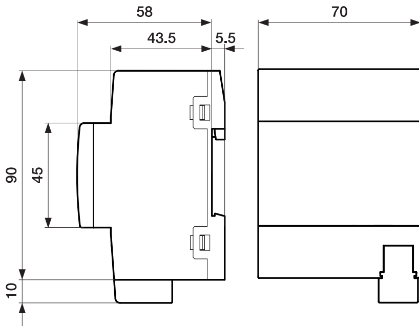
Fig. 5: Plan coté
