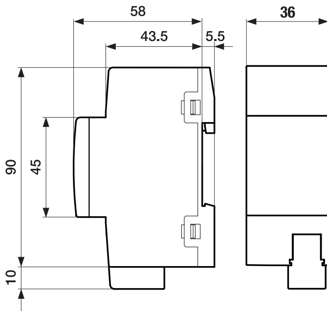
Fig. 2: Plan coté
