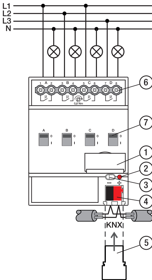
Fig. 6: Schéma de raccordement SA/S 4.x.x.2
