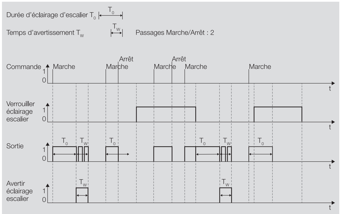
Fig. 19: Comportement Marche-Arrêt de la fonction Éclairage escalier
