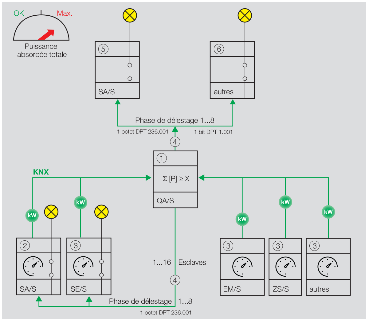
Fig. 15: Le maître ajoute les valeurs de puissance reçues.
