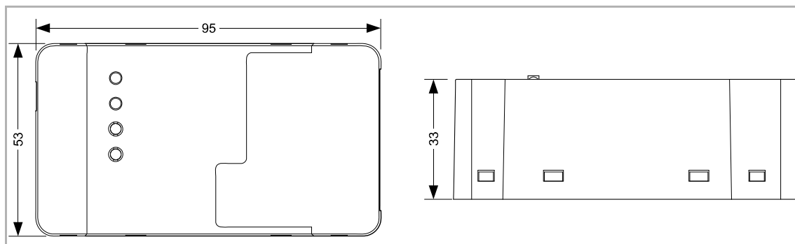
Fig. 3 : Dimensions (toutes les cotes en mm)
