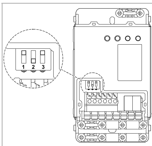
Fig. 7 : commutateur DIP
